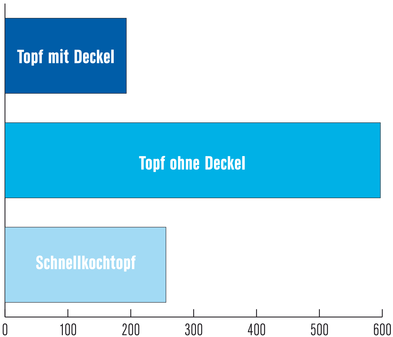
Energieverbrauch zum Garen von 1 kg Pellkartoffeln in Wh
